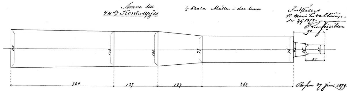
Ritning till Bofors första eldrörsgöt 1879
